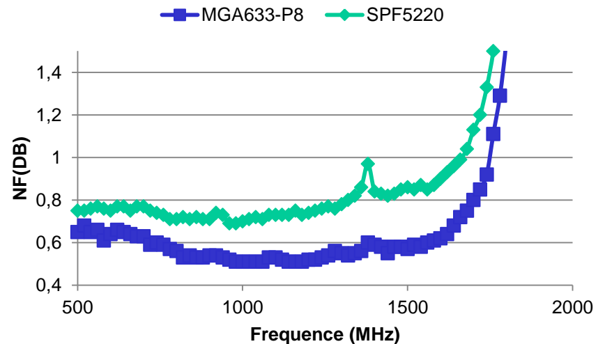
NF(F) LNA_Parabole
