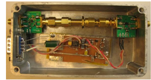
NF(F) LNA_Parabole
