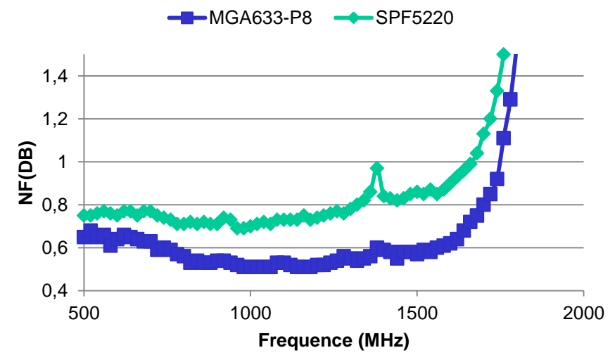
NF(F) LNA_Parabole
