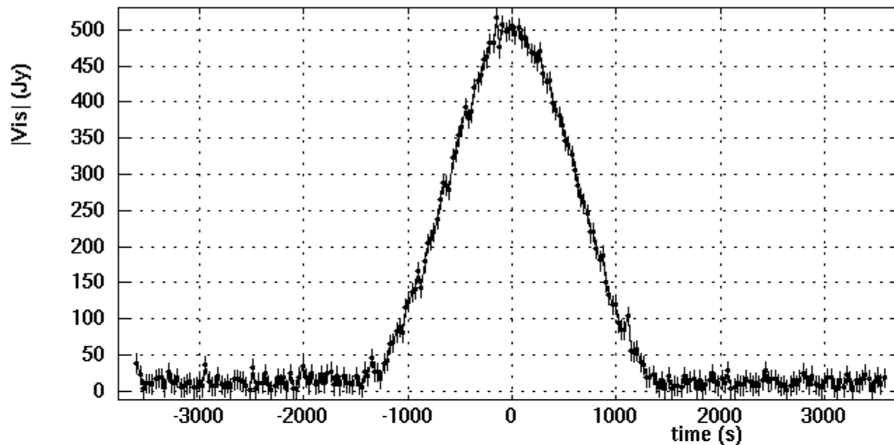
500 Jy - noise 10 Jy - NS tilt 1 m
