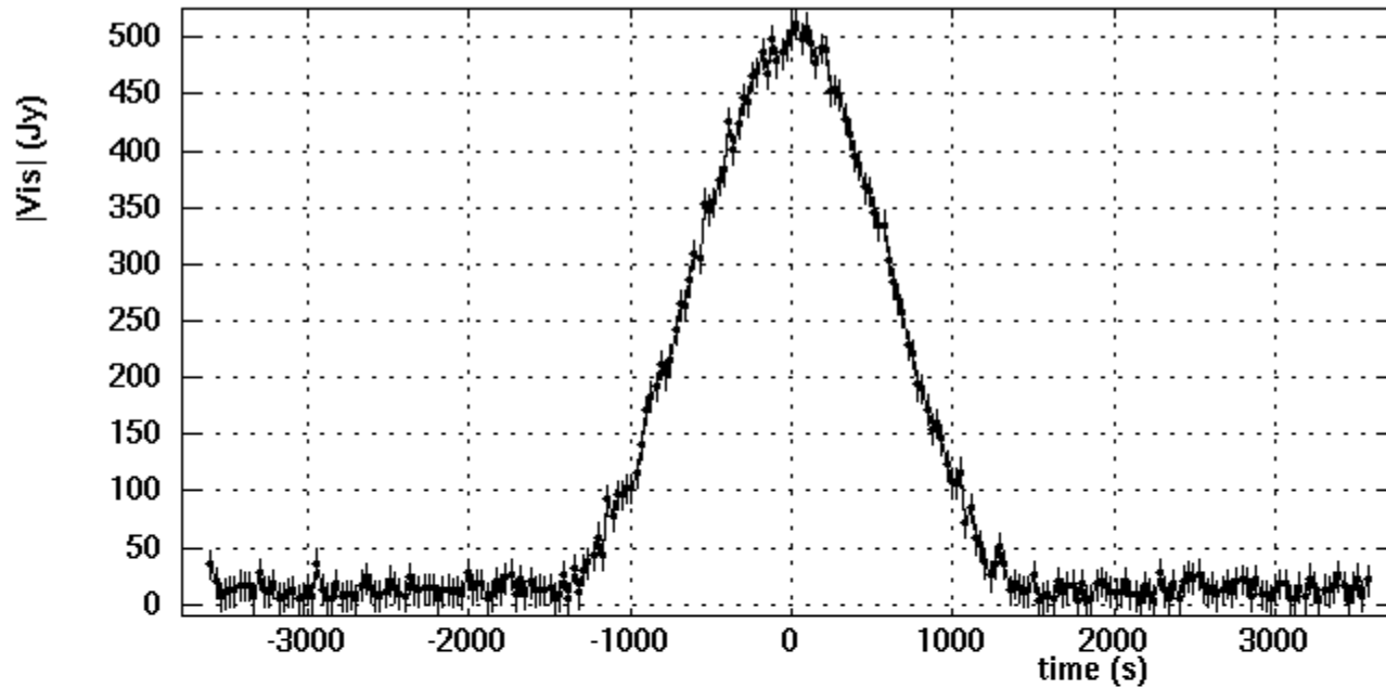
500 Jy - noise 10 Jy - NS tilt 2 m
